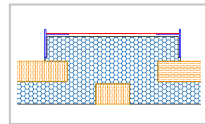
2 Fascia centrale da rasare. Con rete porta intonaco
